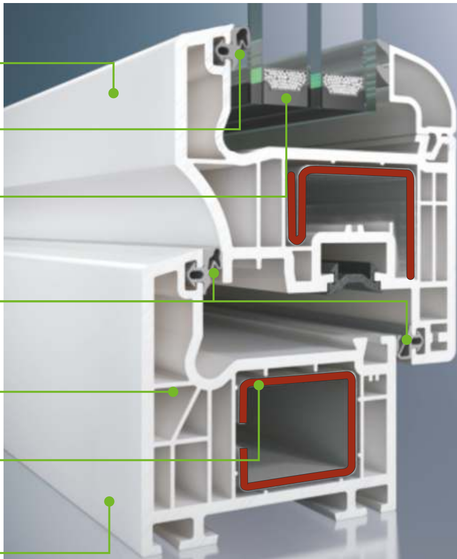
Profil okienny Corona CT 70 Cava
